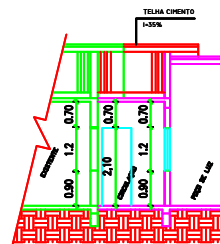
CORTE DD Esc.:1:50
