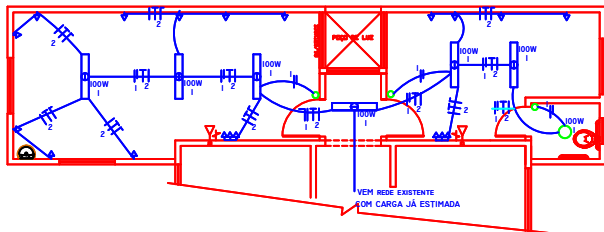
PLANTA BAIXA – ELÉTRICO Esc.:1:50
