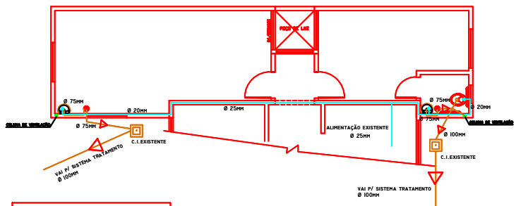
PLANTA BAIXA – HIDROSSANITÁRIO Esc.:1:50
