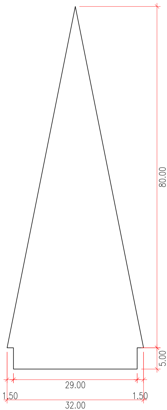
PLANTA DETALHADA DA PONTEIRA MACIÇA DA GRADE FRONTAL Escala: 1:100
