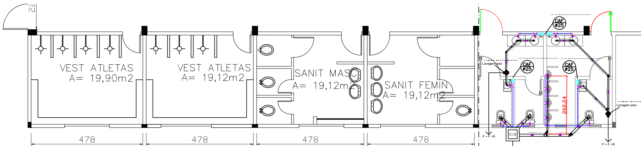
Planta Baixa Hidrossanitário
