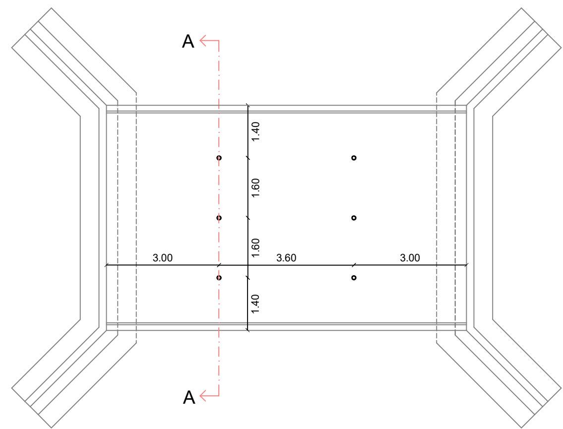
Projeto de Drenagem - Localização dos furos Esc.: 1:100
