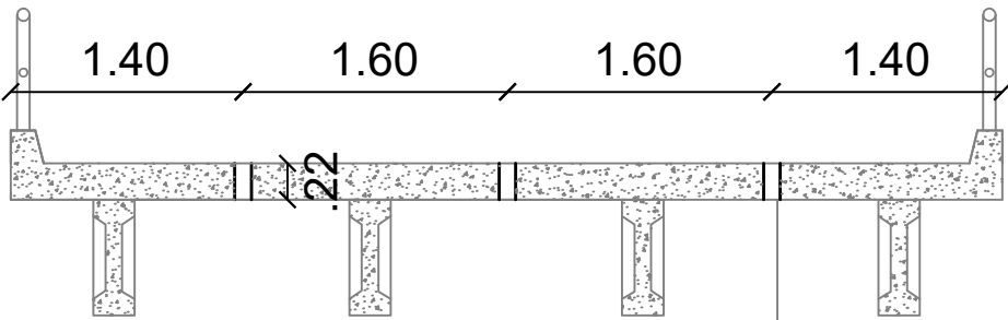
Corte A-A' Esc.: 1:50 Tubo de PVC DN 100 mm
