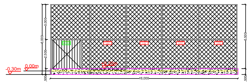
VISTA 04 ESC. 1:100
