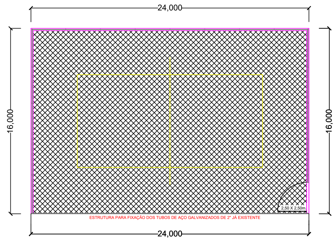
PLANTA BAIXA REDE DE NYLON PARA COBERTURA ESC. 1:100
