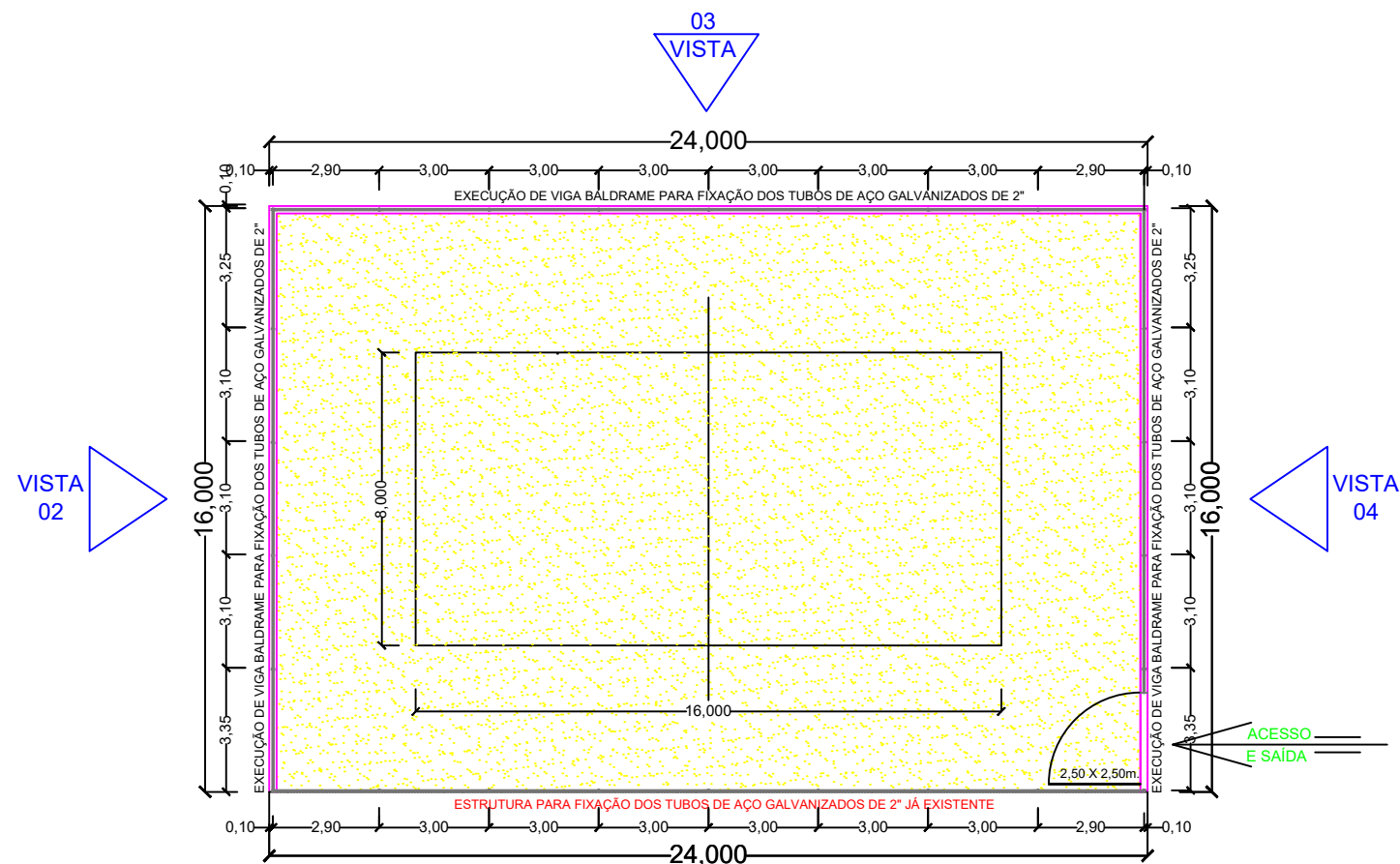
PLANTA BAIXA ALAMBRADO ESC. 1:100
