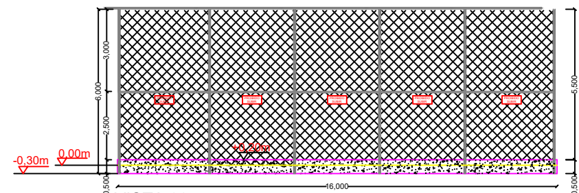
VISTA 02 ESC. 1:100
